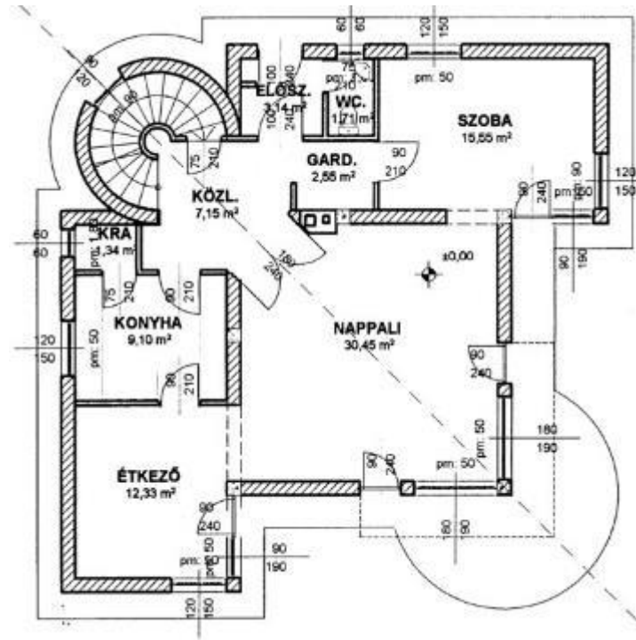
földszint
