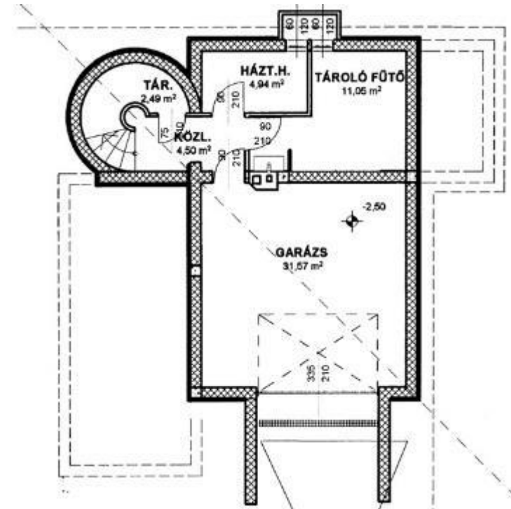
pinceszint
